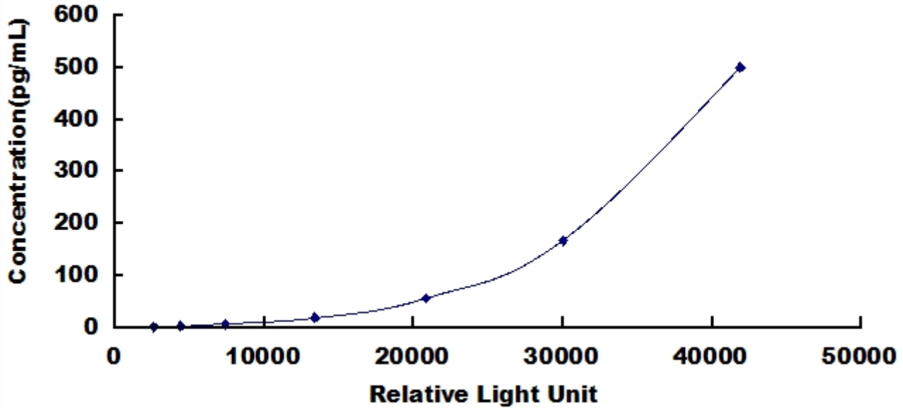
人白介素 6 (IL6) 检测试剂盒标准曲线
