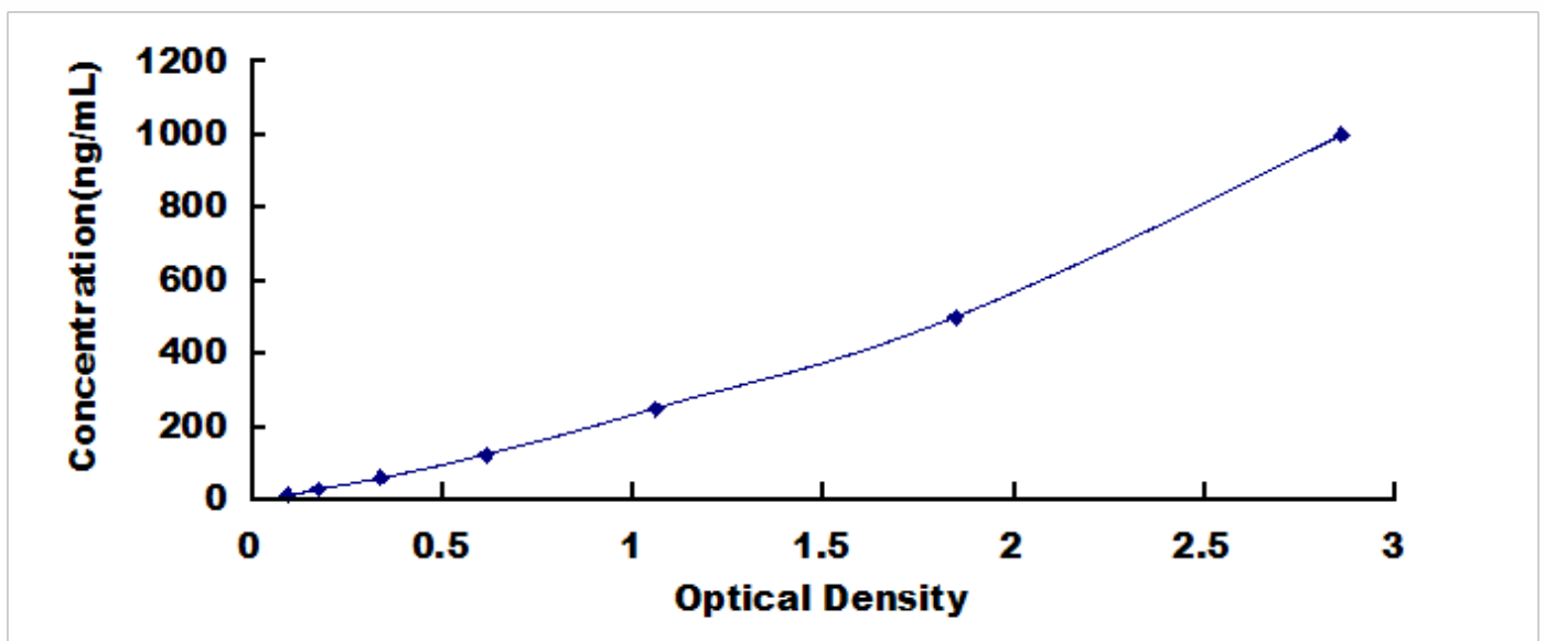
牛 \alpha 1-酸性糖蛋白 ( \alpha 1AGP) 检测试剂盒标准曲线
