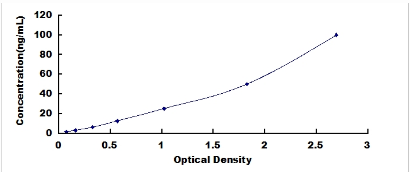
牛 \alpha -乳清蛋白 ( \alpha LA) 检测试剂盒标准曲线
