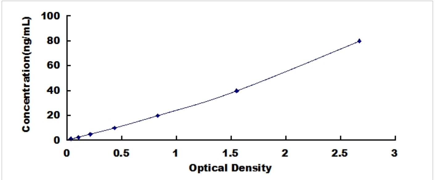
小鼠载脂蛋白 C1 (APOC1) 检测试剂盒标准曲线
