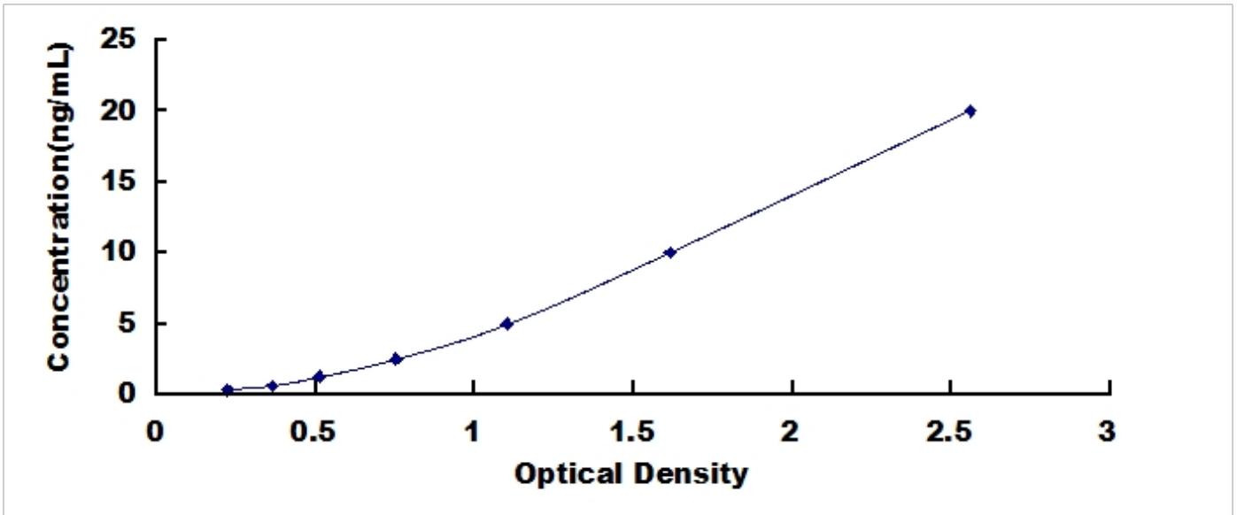
人芳香烃受体核转位因子样蛋白 (ARNTL) 检测试剂盒标准曲线
