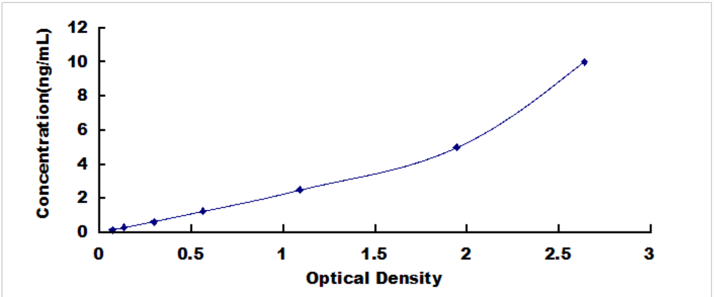
大鼠 BMP 结合内皮调节因子(BMPER)检测试剂盒标准曲线
