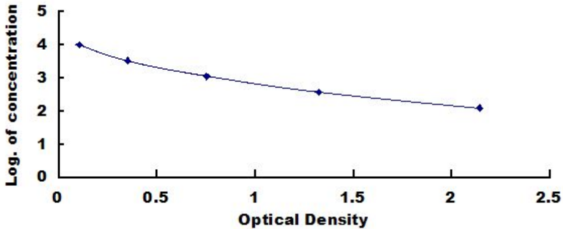
小鼠β2-微球蛋白(b2M)检测试剂盒标准曲线
