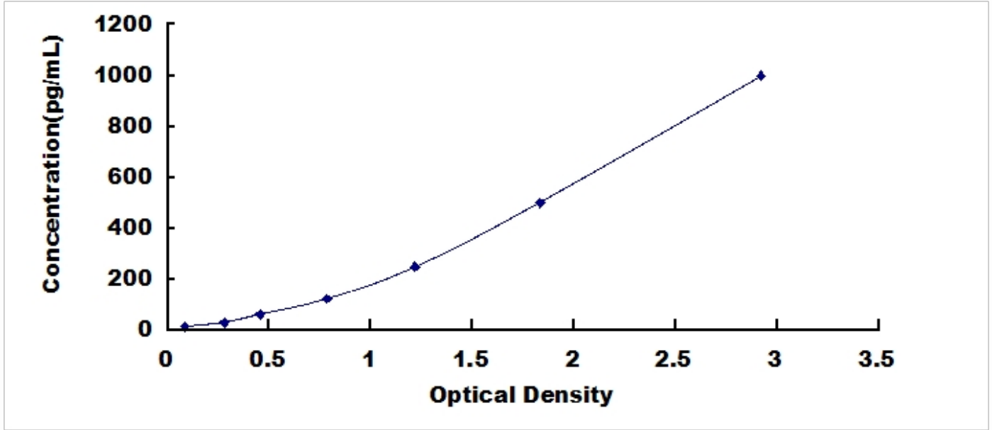
人碳酸酐酶XII (CA12) 检测试剂盒标准曲线
