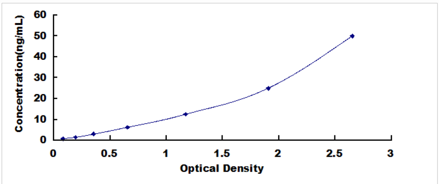
小鼠 18kDa 阳离子抗菌肽 (CAMP) 检测试剂盒标准曲线
