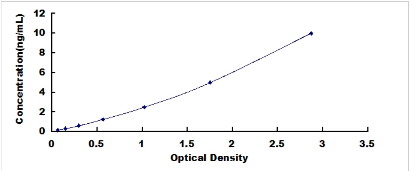
人 L1CAM 同源物细胞粘附分子(CHL1)检测试剂盒标准曲线
