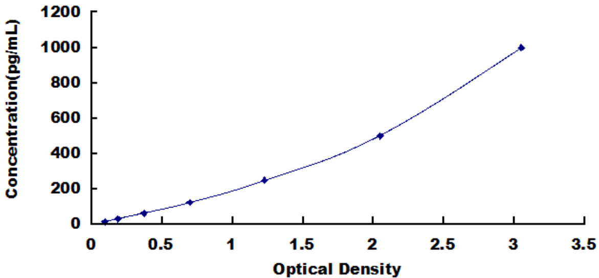
小鼠淋巴细胞趋化因子(Lptn)检测试剂盒标准曲线
