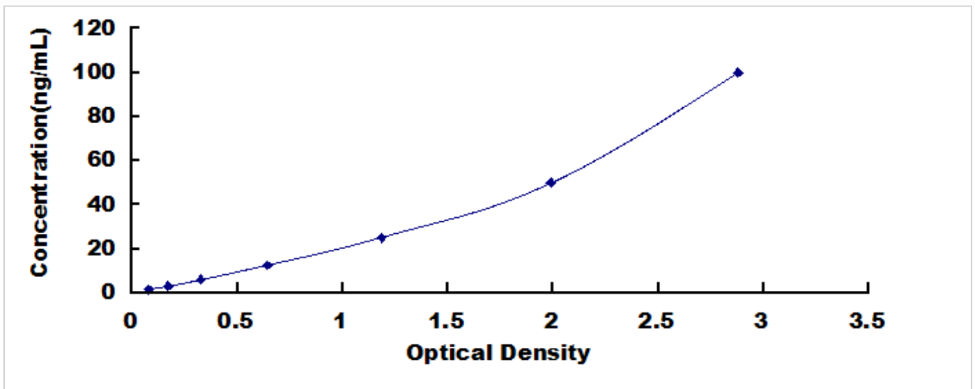
大鼠细胞色素 P450 家族成员 2D6 (CYP2D6) 检测试剂盒标准曲线
