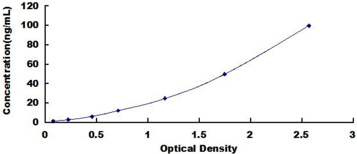
人细胞色素 P450 家族成员 4F2 (CYP4F2) 检测试剂盒标准曲线
