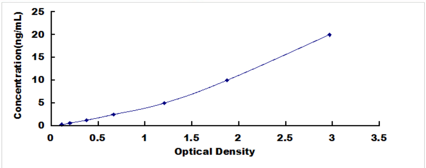
人细胞角蛋白 19 片段抗原 21-1 (CYFRA21-1) 检测试剂盒标准曲线
