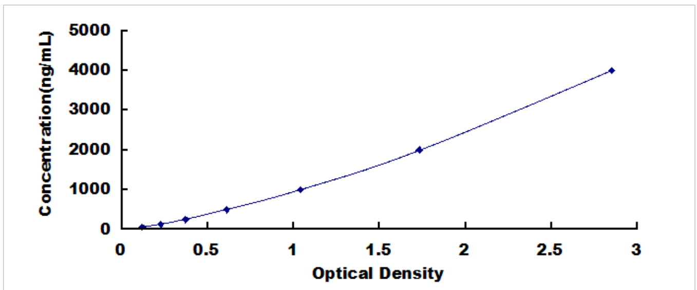
大鼠纤维蛋白原 (FG) 检测试剂盒标准曲线
