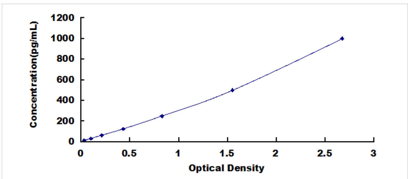
大鼠磷脂酰肌醇蛋白聚糖 4 (GPC4) 检测试剂盒标准曲线
