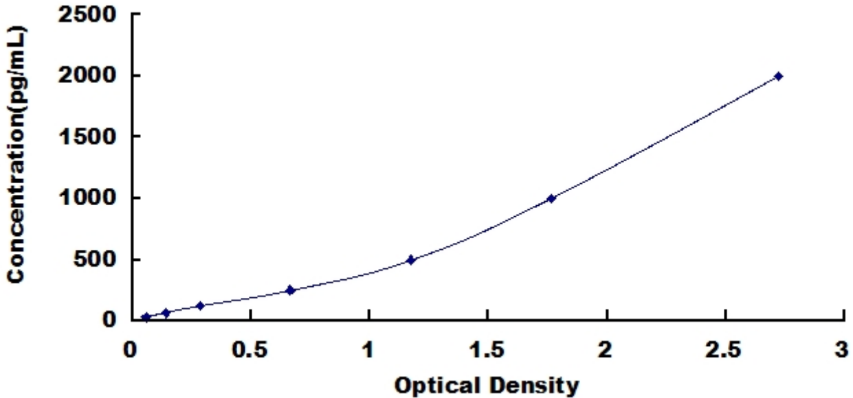
小鼠颗粒体蛋白 (GRN) 检测试剂盒标准曲线
