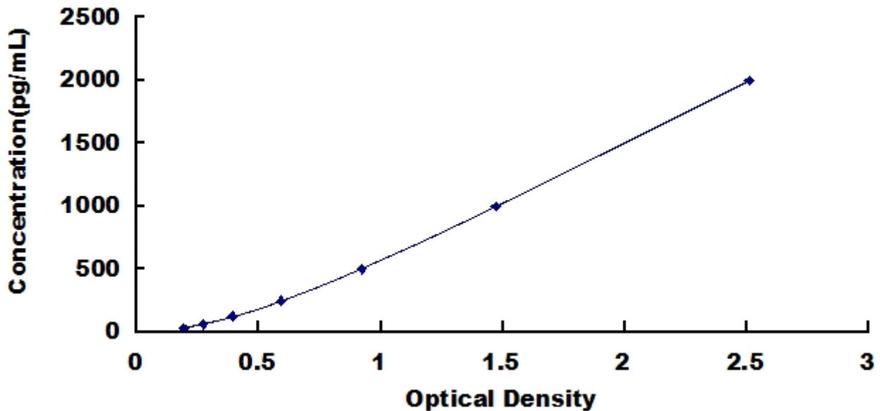
人整合素连接激酶（ILK）检测试剂盒标准曲线
