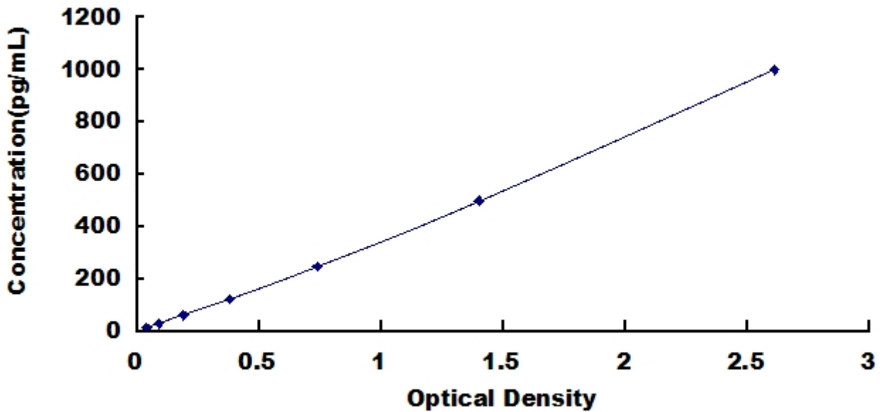
小鼠干扰素 \gamma 诱导单核因子(MI \gamma ) 检测试剂盒标准曲线
