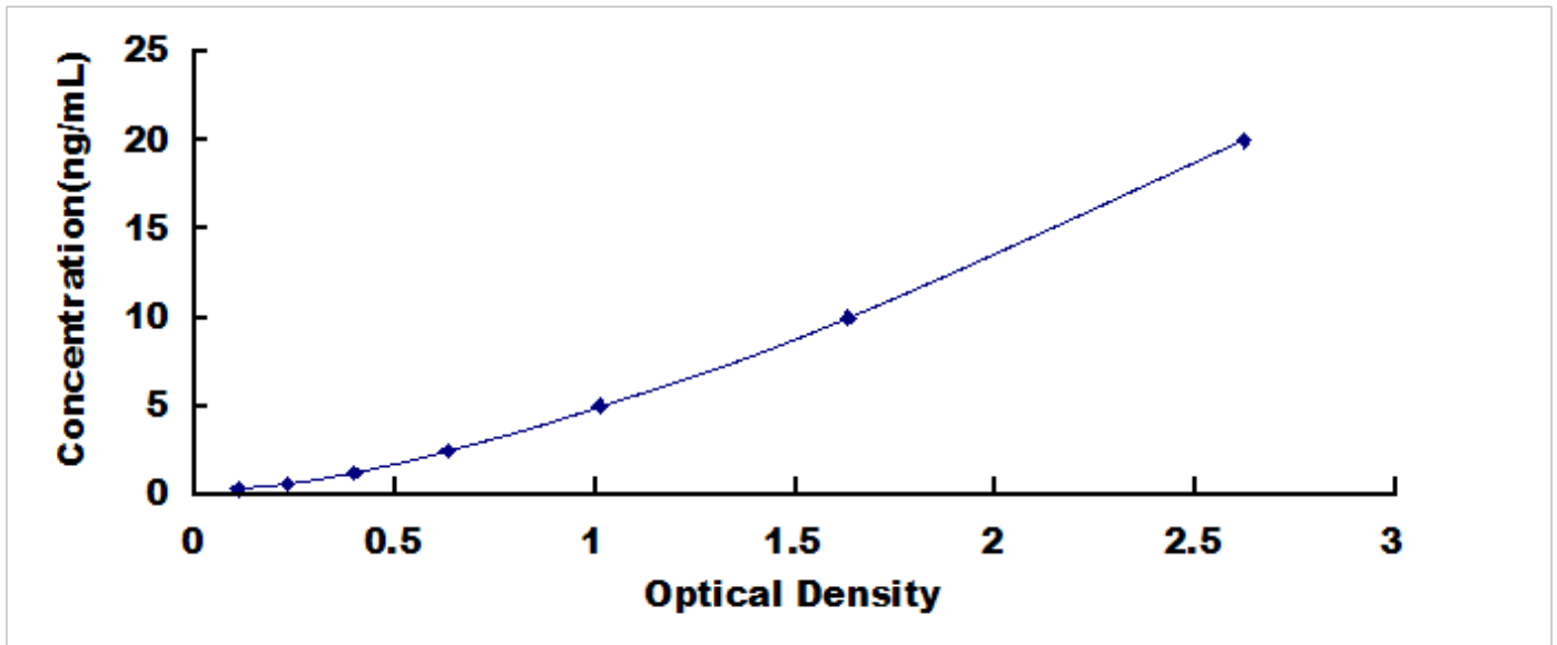
人 N-酰基乙醇氨酸酰化酶 (NAAA) 检测试剂盒标准曲线
