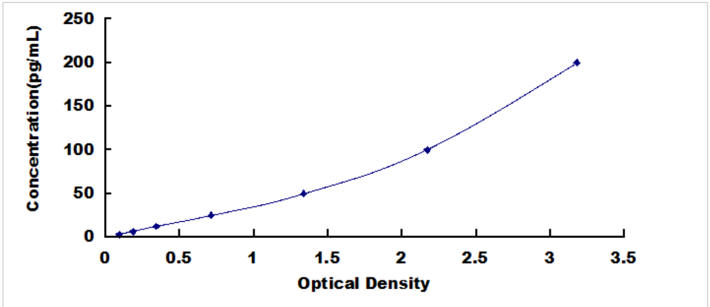
大鼠神经营养因子 3 (NT3) 检测试剂盒标准曲线
