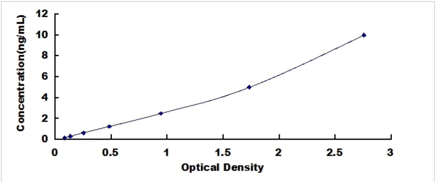
大鼠围脂滴蛋白 3 (PLIN3) 检测试剂盒标准曲线
