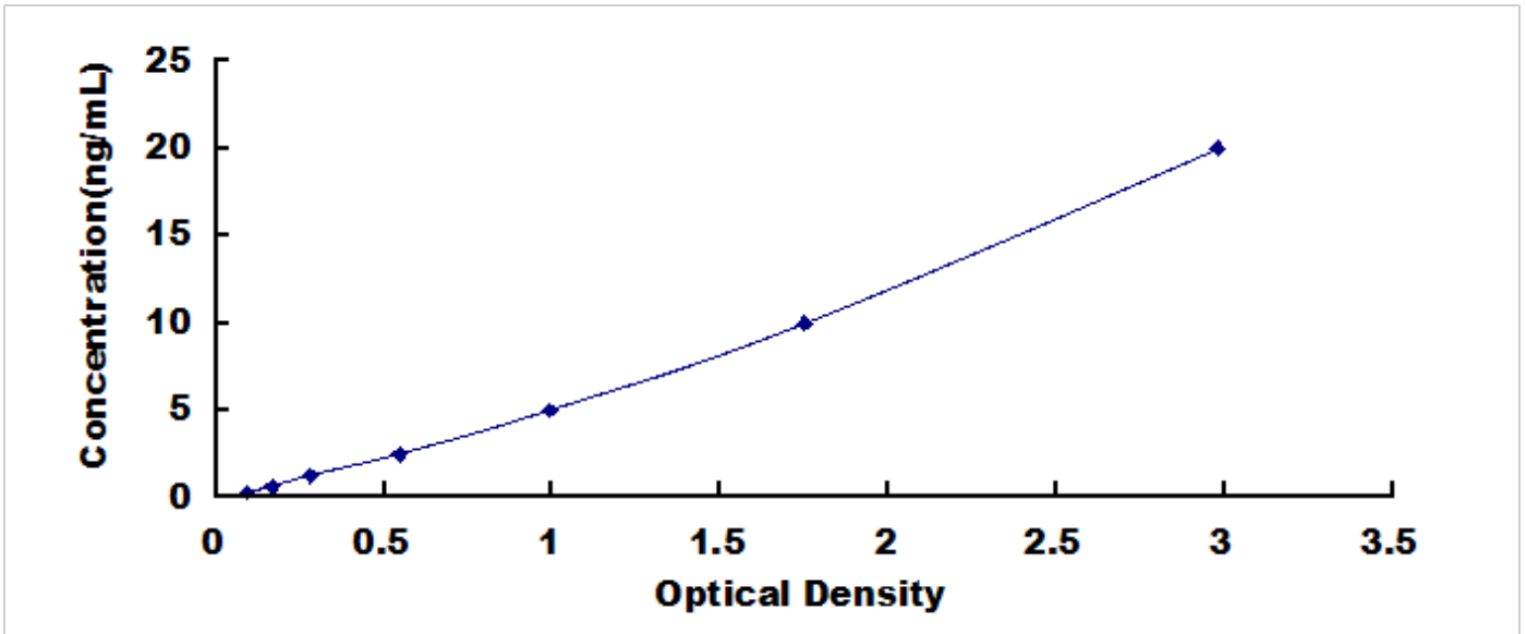
大鼠过氧化物酶体增殖物激活受体 \alpha (PPAR \alpha ) 检测试剂盒标准曲线
