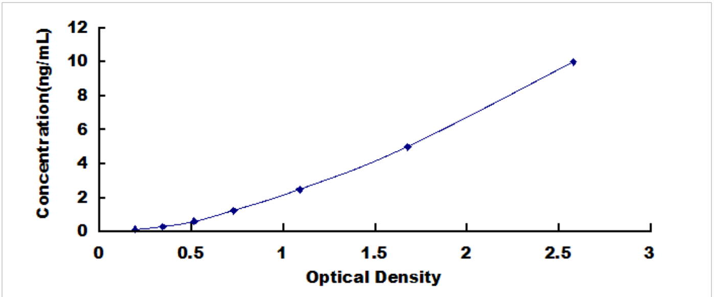
人 DNA 指导聚合酶 β (POL β) 检测试剂盒标准曲线
