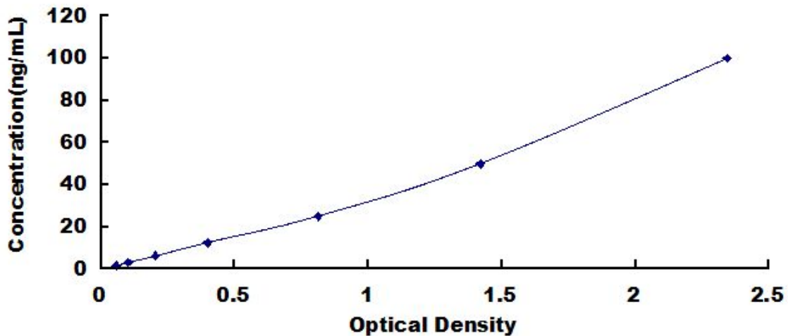
大鼠肾酶(RNLs)检测试剂盒标准曲线
