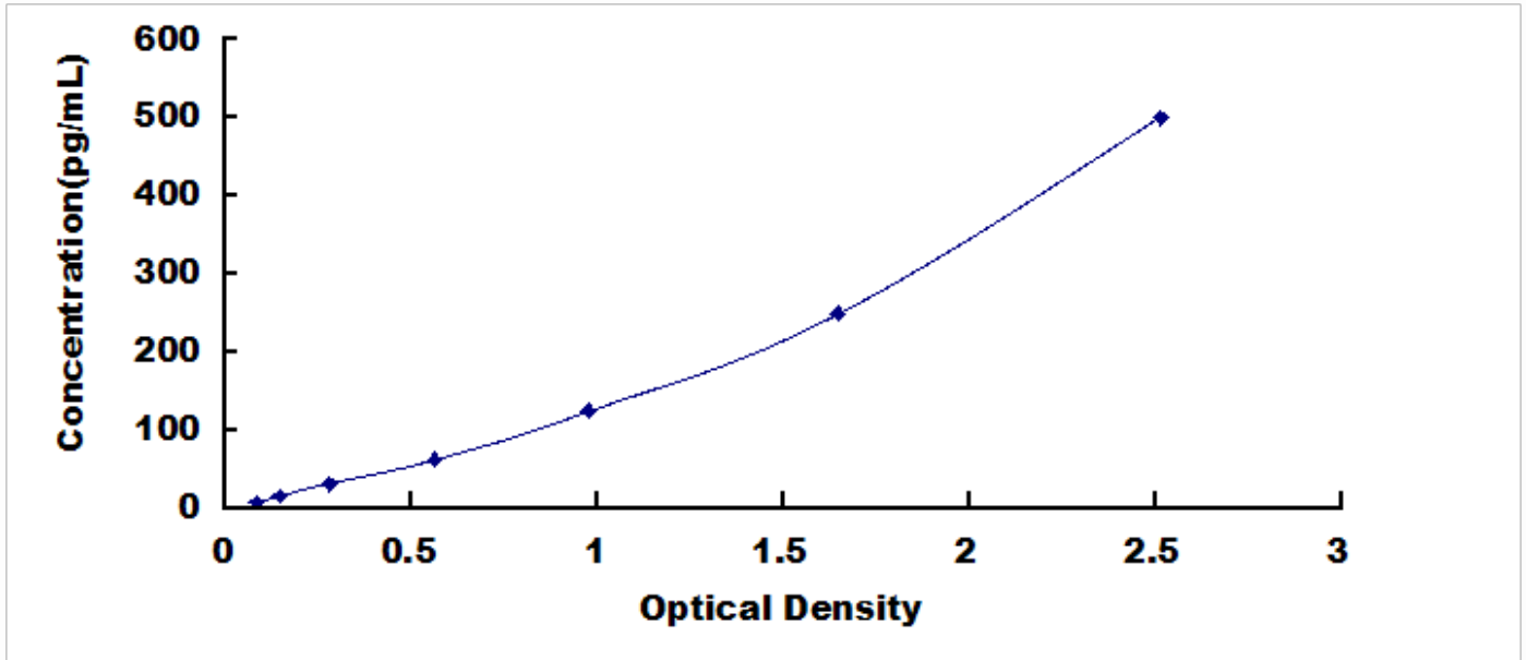
小鼠血小板生成素 (TPO) 检测试剂盒标准曲线
