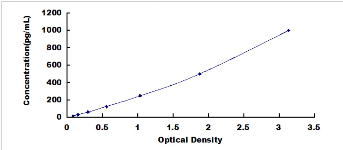
兔心肌肌钙蛋白 I (TNNI3) 检测试剂盒标准曲线
