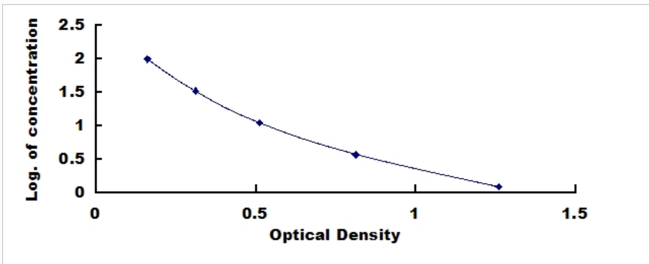
色氨酸(Trp)检测试剂盒标准曲线
