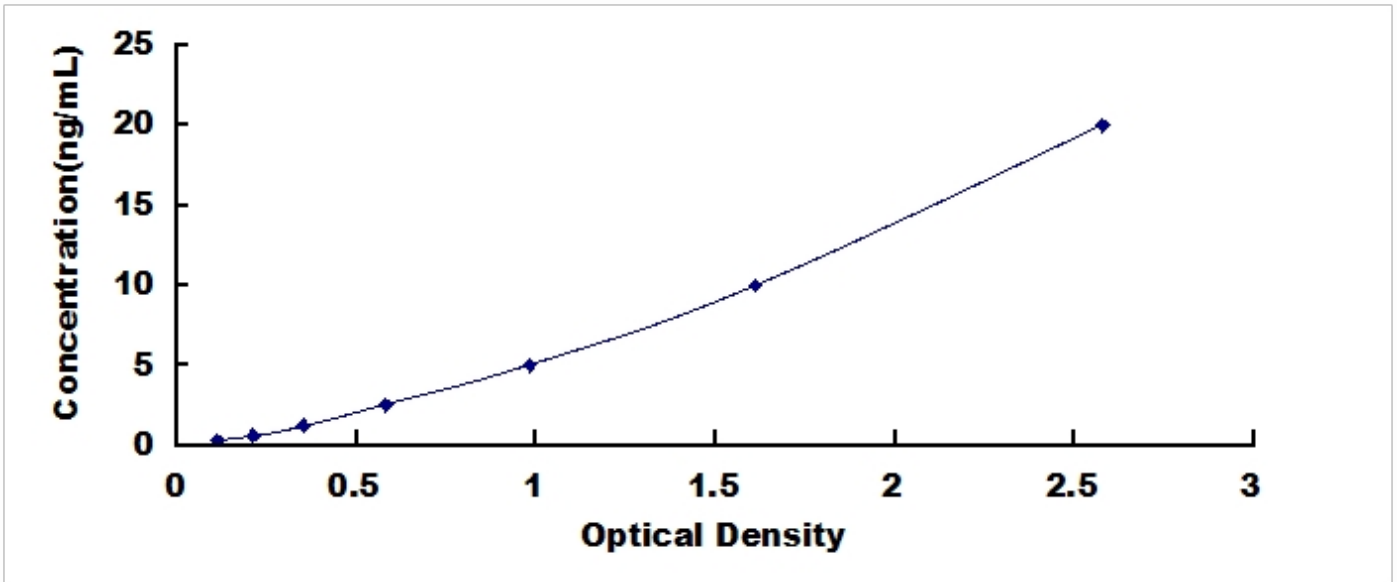
小鼠翻译调节肿瘤蛋白 1 (TPT1) 检测试剂盒标准曲线
