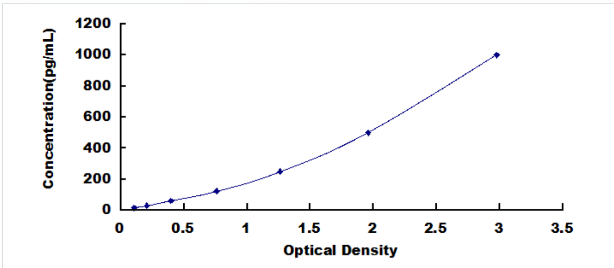
犬血管内皮生长因子 A (VEGFA) 检测试剂盒标准曲线
