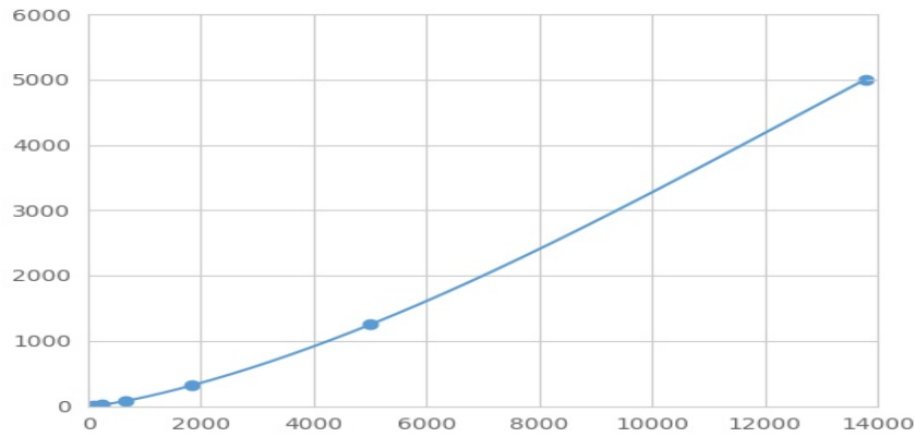
(解整合素金属蛋白酶8)检测试剂盒标准曲线
