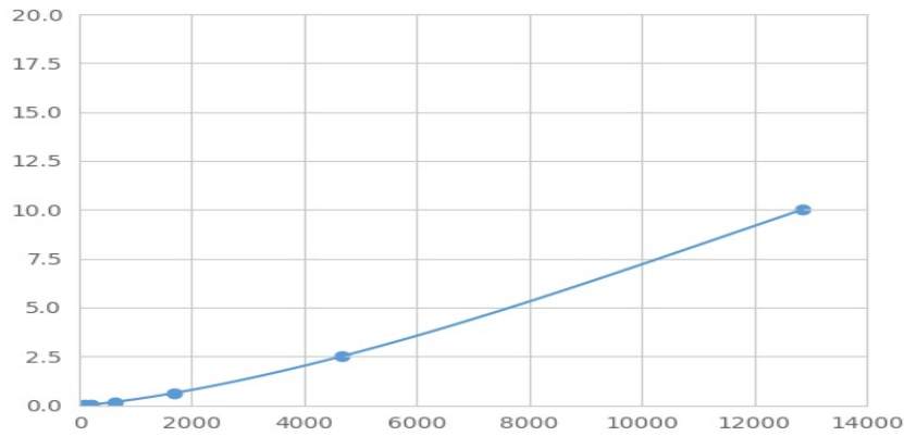
(ATP结合盒转运蛋白C13)检测试剂盒标准曲线
