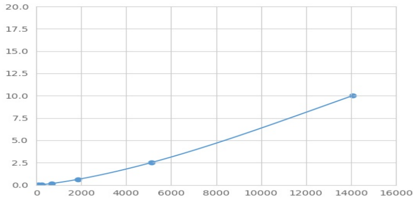
(钠/钾离子转运ATP酶β 4肽)检测试剂盒标准曲线
