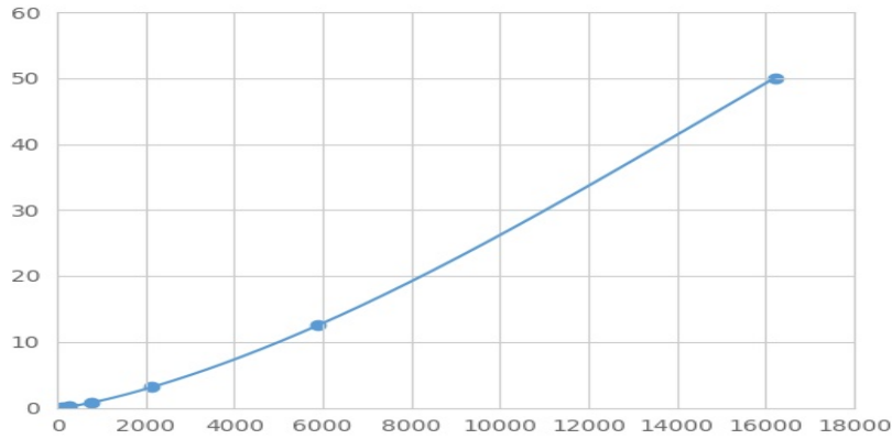
(乙醇脱氢酶4)检测试剂盒标准曲线
