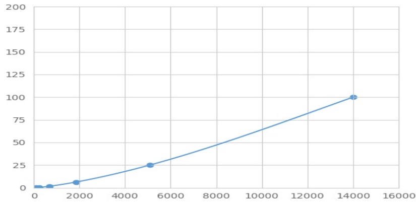
(果糖二磷酸醛缩酶A)检测试剂盒标准曲线
