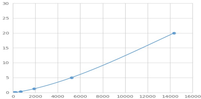
(B-细胞淋巴瘤因子9样蛋白)检测试剂盒标准曲线
