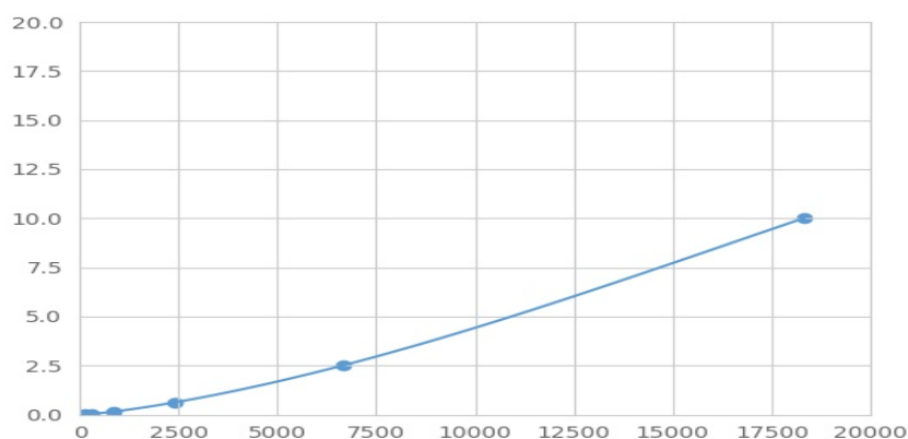
(C4结合蛋白 α) 检测试剂盒标准曲线
