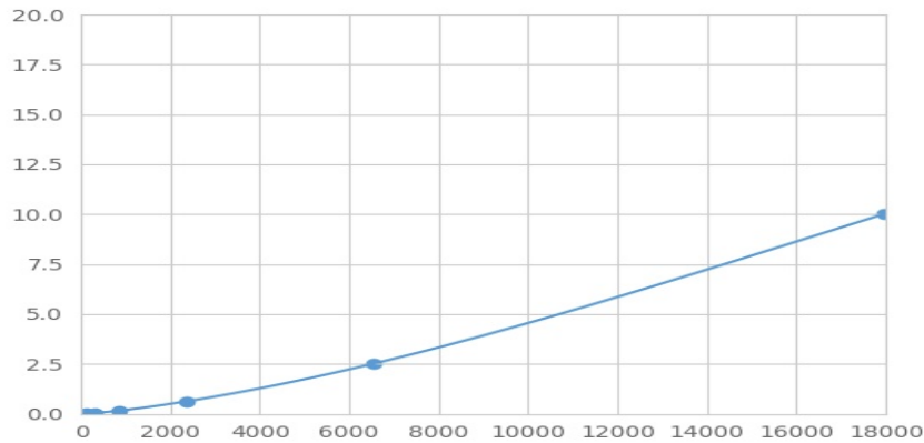
(连环蛋白 α 1) 检测试剂盒标准曲线
