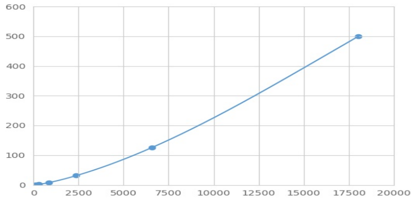
(结缔组织生长因子)检测试剂盒标准曲线
