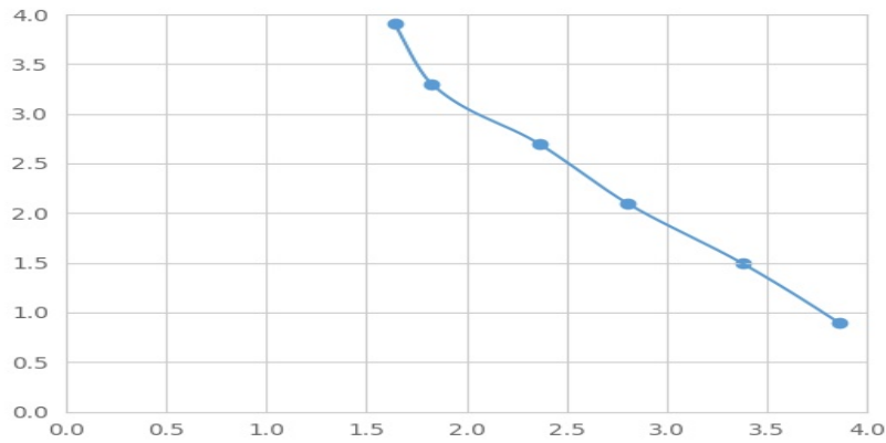
(II型胶原交联羧基端肽)检测试剂盒标准曲线
