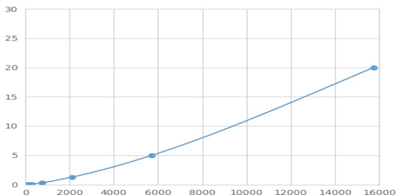
(细胞色素C氧化酶亚基III)检测试剂盒标准曲线
