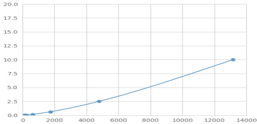
(细胞色素P450家族成员11B1)检测试剂盒标准曲线
