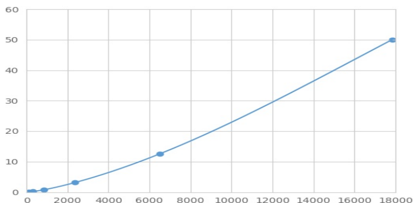
(碘甲腺原氨酸脱碘酶 II) 检测试剂盒标准曲线
