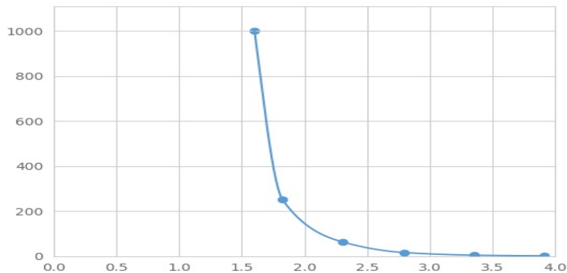
(多巴胺)检测试剂盒标准曲线
