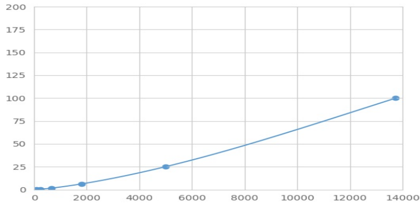
(丝织蛋白样蛋白)检测试剂盒标准曲线
