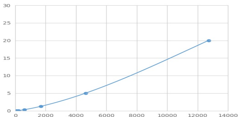
(双丝氨酸/苏氨酸酪氨酸蛋白激酶)检测试剂盒标准曲线
