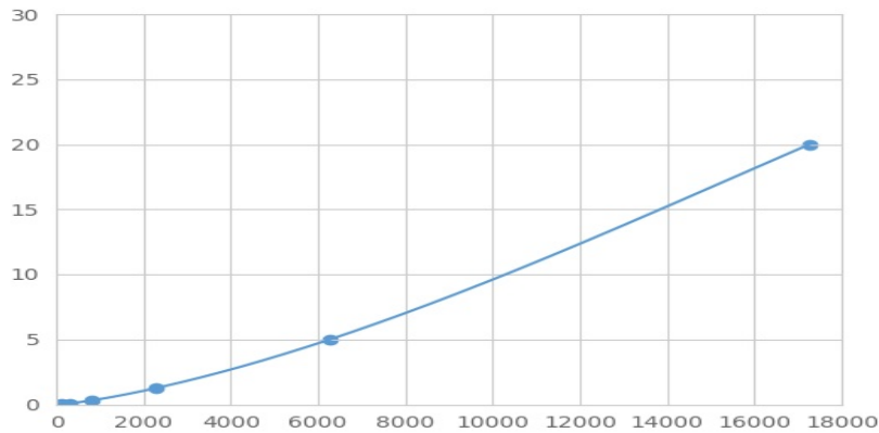
(肌动蛋白束蛋白)检测试剂盒标准曲线
