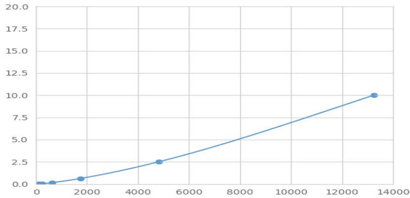
(G蛋白 \alpha 转导活性多肽1)检测试剂盒标准曲线
