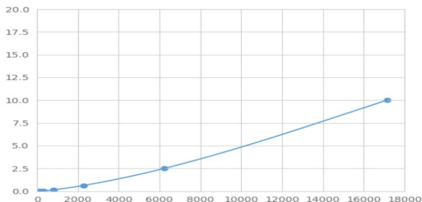
(半乳糖-1-磷酸尿苷酰转移酶)检测试剂盒标准曲线
