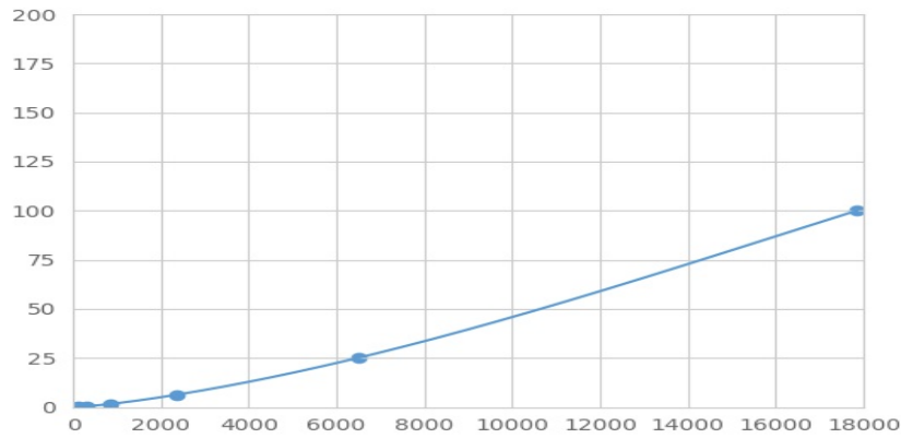
(线粒体甘油-3-磷酸酰基转移酶)检测试剂盒标准曲线
